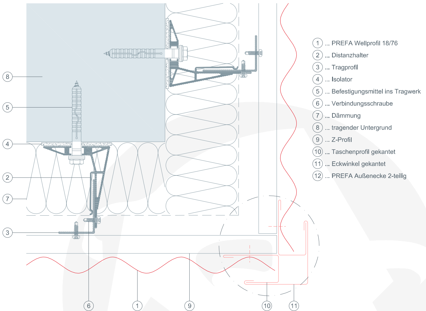
Anschlussvariante
